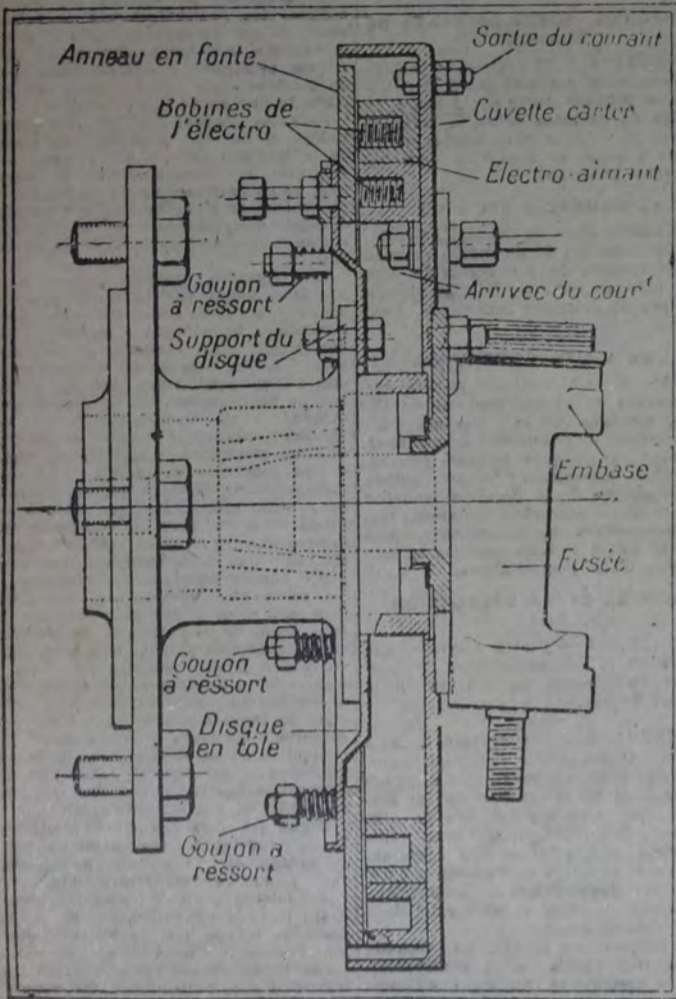
Corte del freno electromagnético
