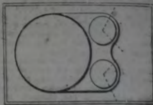
Fig. 2. Mala forma de culata. Las válvulas están demasiado próximas a la pared del cilindro, por lo que una tercera de su circunferencia se encuentra inutilizada.
