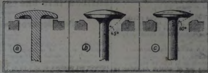
Fig. 1. Diversas formas de válvulas: a) válvula a asiento plano; b) válvula a 45°; c) válvula a 60°.
