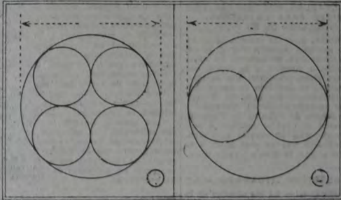
Fig. 2. Disposición esquemática de válvulas colocadas en el fondo de la culata de un cilindro de un diámetro dado d. a) en caso de dos válvulas. La circunferencia de cada válvula es como máximo igual a 0,5 n d. b) en caso de cuatro válvulas. La circunferencia total de las dos válvulas es igual a 0,53 n d. o sea una ganancia de 49 por 100 con respecto al caso de dos válvulas.
