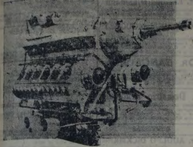
El motor "Farman" invertido, 18 cilindros (110 x 125 mm.)
